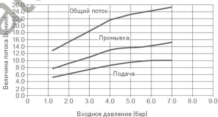
ИНЖЕКТОР 5С
