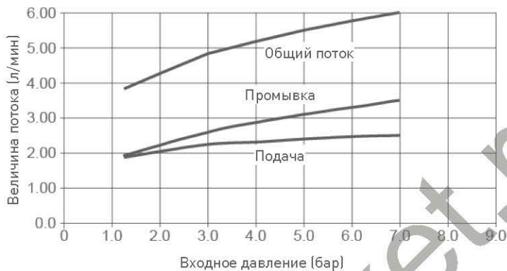
ИНЖЕКТОР 2
