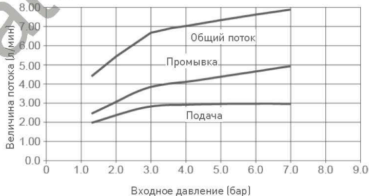
ИНЖЕКТОР 3
